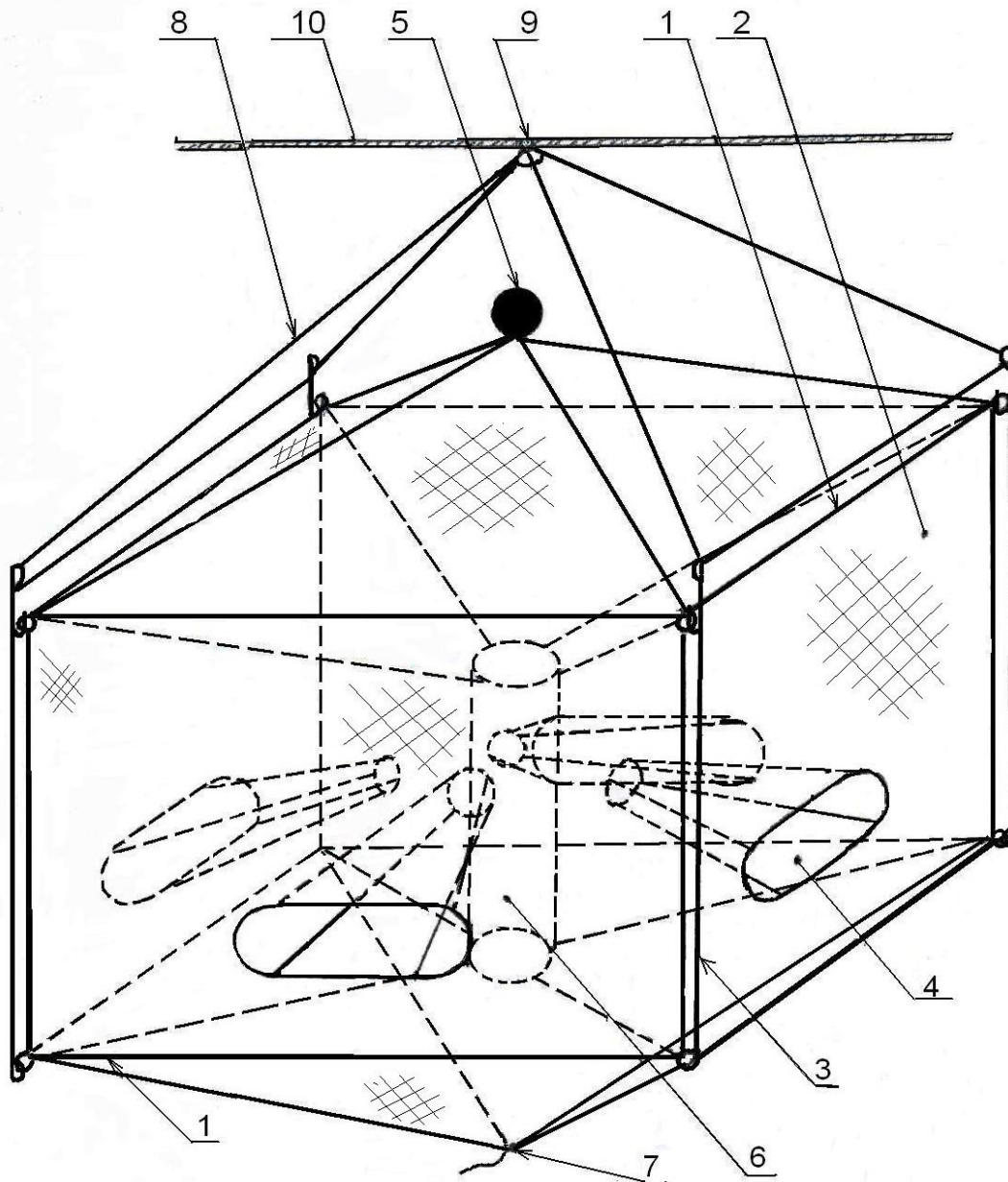
Рисунок 4 – Подъемная ловушки: 1 – нижний и верхний каркасы; 2 – сетная часть; 3 – стойка; 4 – входа; 5 – поплавок; 6 – приманка; 7 – распускное отверстие; 8 – усы; 9 – скоба с карабином; 10 – вожак
