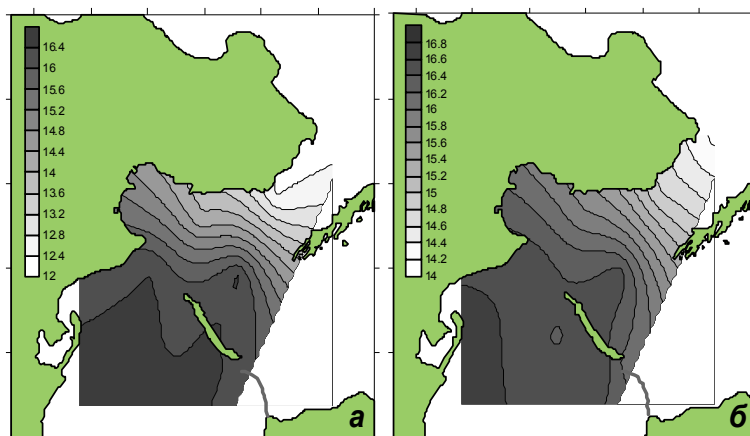
Рисунок 2 – Распределение солености (‰) в поверхностном (а) и придонном (б) горизонтах вод
