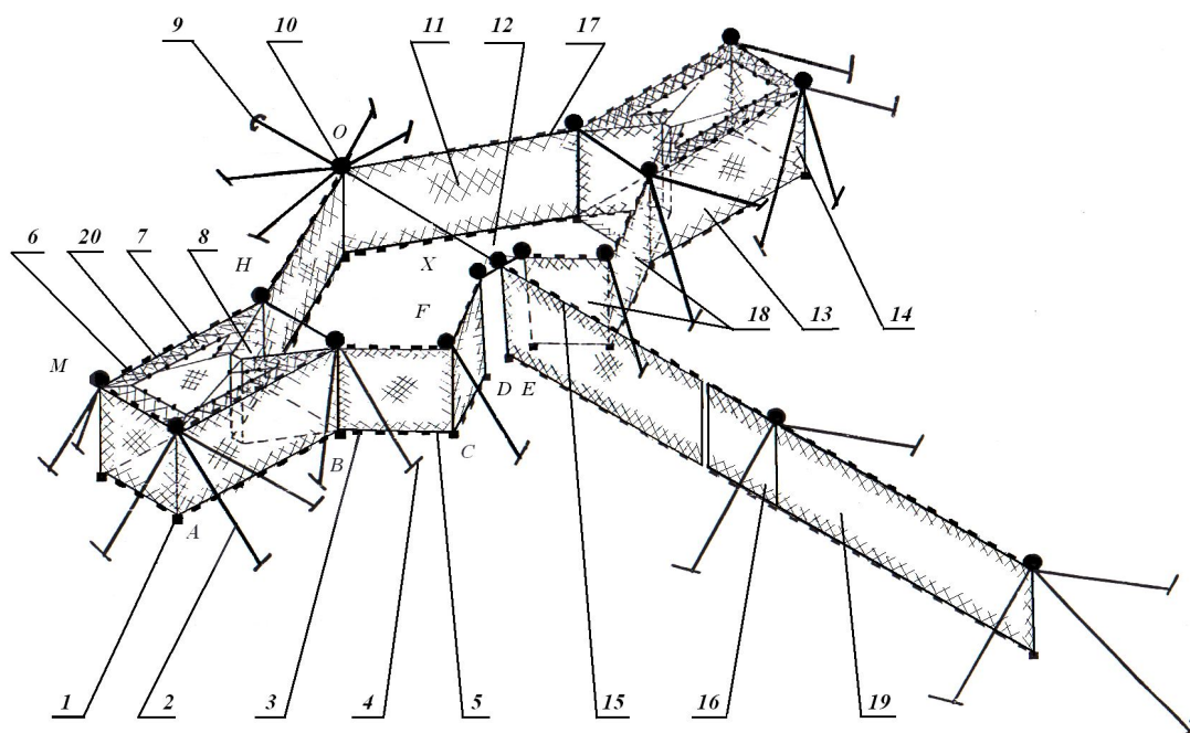
Рисунок 1 – Невод ставной штормоустойчевый: 1 – угловой груз; 2 – наклонная оттяжка; 3 – груз распределенной загрузки; 4 – кол; 5 – нижняя подбора; 6 – поплавок; 7 – козырек; 8 – усынок; 9 – якорь; 10 – угловой буй; 11 – морская стенка; 12 – двор ловушки; 13 – котел; 14 – сливная стенка; 15 – становой трос; 16 – направляющее крыло; 17 – верхняя подбора; 18 – открылок; 19 – дель (сетное полотно); 20 – рама
